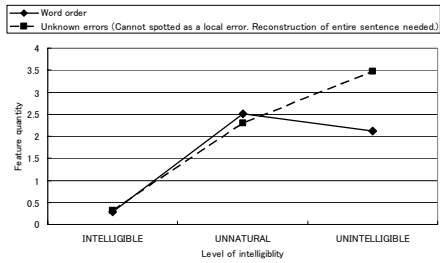
Fig. 8. Global Errors
